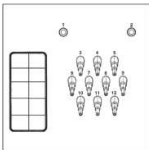
Přípojky dávkovacích čerpadel na zadní straně přístroje
