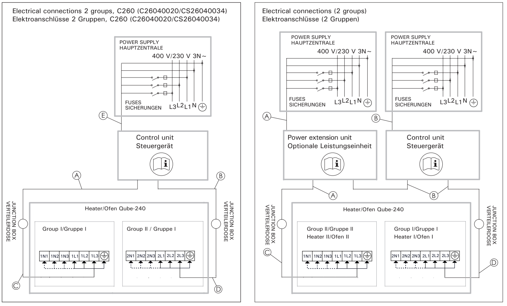
Figure 10. Abbildung 10. Electrical connections of control unit and heater Elektroanschlüsse des Steuergerät und des Saunaofens
