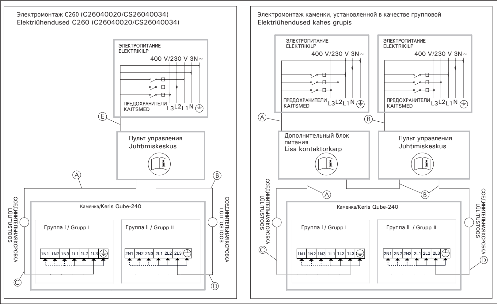
Рисунок 9. Электромонтаж пульта управления и каменки Joonis 9. Juhtimiskeskuse kütise
