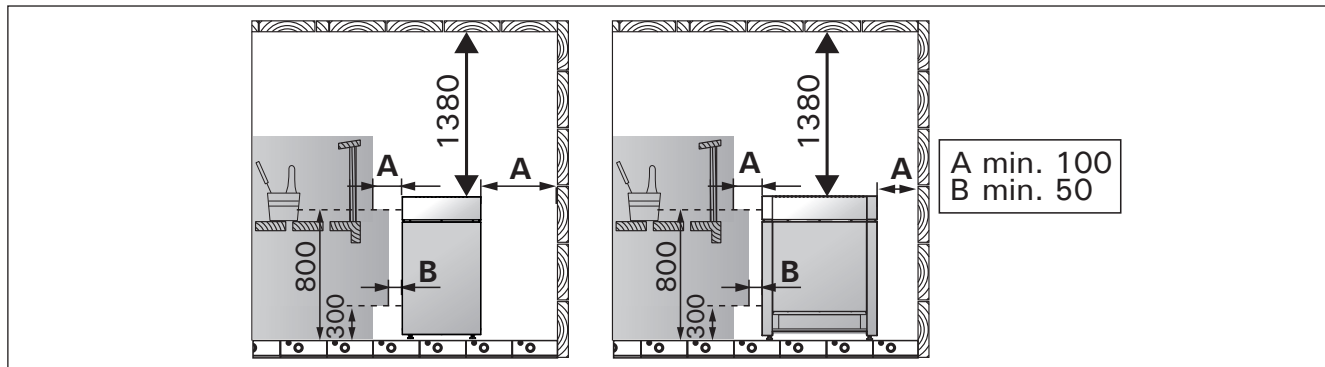
Рисунок 4. Расстояния безопасности (все размеры приведены в миллиметрах) Joonis 4. Kerise ohutuskaugetused (kõik mõõtmised millimeetrites)
