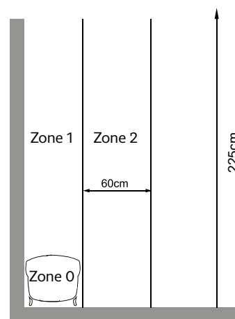
Seitensicht Badewanne
