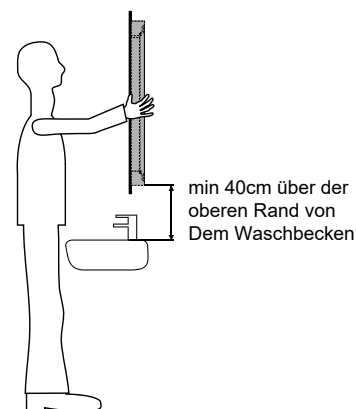
Seitensicht Waschbecken
