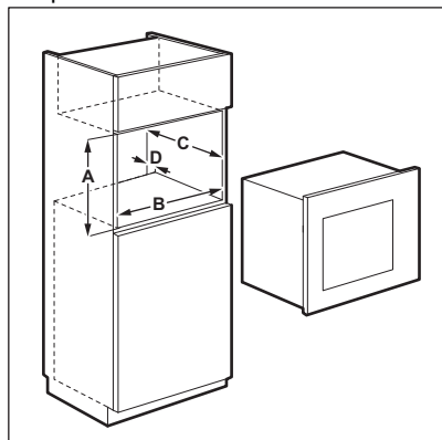
Montážne vzdialenosti
