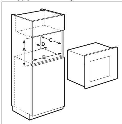
Monteringsavstånd
