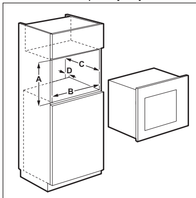
Монтажни растојанија
