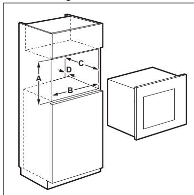
Monteringsavstand
