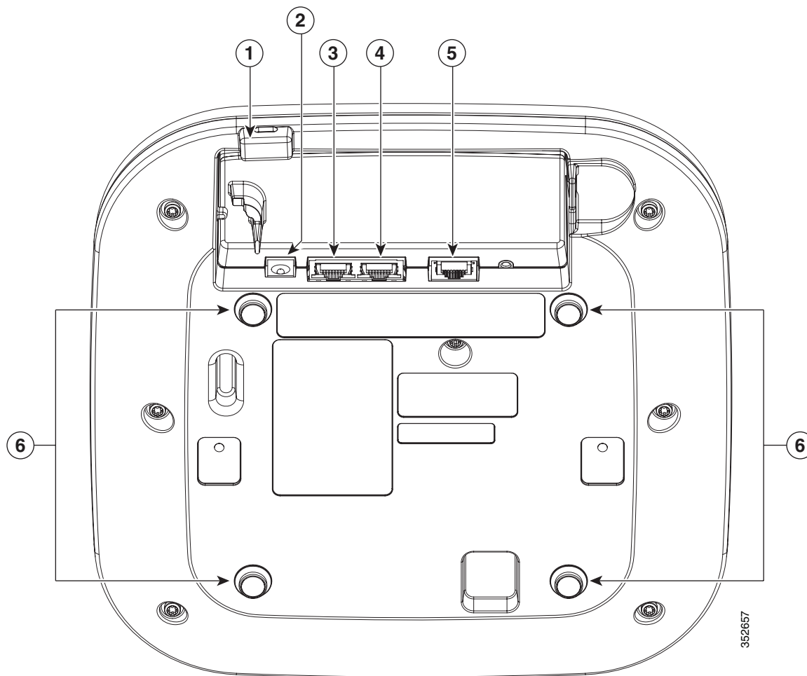
図 3 アクセス ポイントのポートと接続部（下部） - AIR2702E および 2702I モデル
