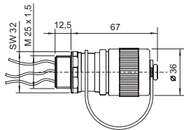
Flange socket (metal)
