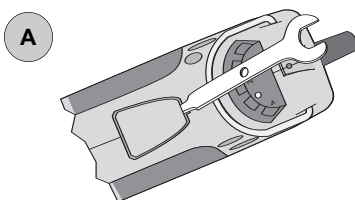
Remoción de la tapa de la cavidad de la escobilla
