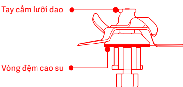
Lưỡi dao xay
