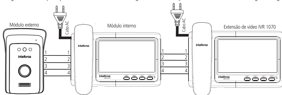
Instalação de extensão de vídeo IVR 1070
