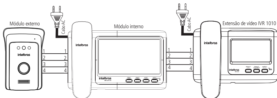
Instalação da extensão de vídeo com o IVR 1010
