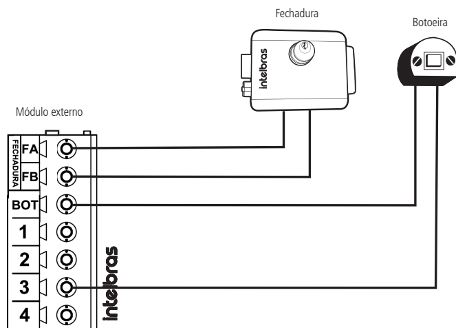
Instalação de fechadura elétrica e botoeira
