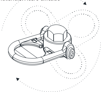
Anclaje basculante de punto único para estructura de concreto (DXFP843101)
