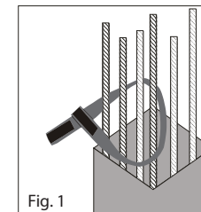
Fig. 1 Avant de bétonner
