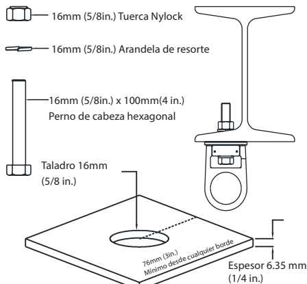
Anclaje basculante de punto único para estructura de Metal (DXFP843102)
