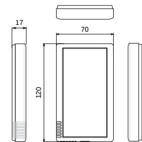
REMOTE SENSOR (CZ-CSRC3)
