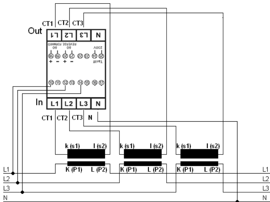
Abb.: Pin-Belegung
