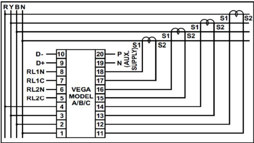
Abb.: Pin-Belegung
