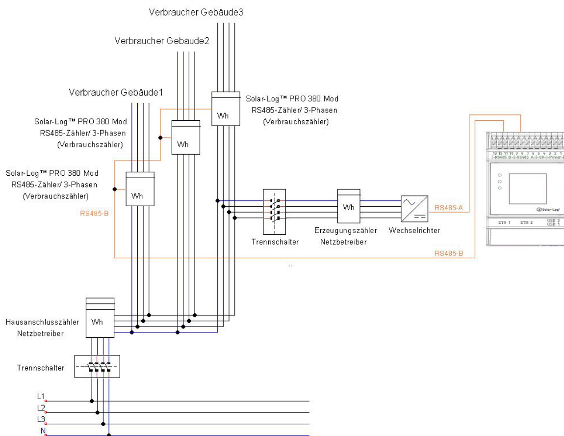
Abb.: Direkte Verbrauchsmessung mit mehreren Zählern
