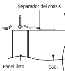
Vista superior
