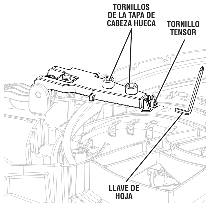
SIERRA VISTA DESDE ABAJO
