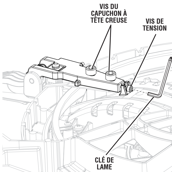
VUE DU DESSOUS DU SCIE
