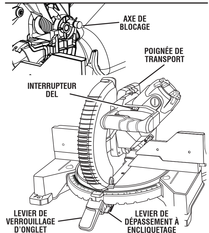
BRAS BLOQUÉ EN POSITION ABAISSÉE
