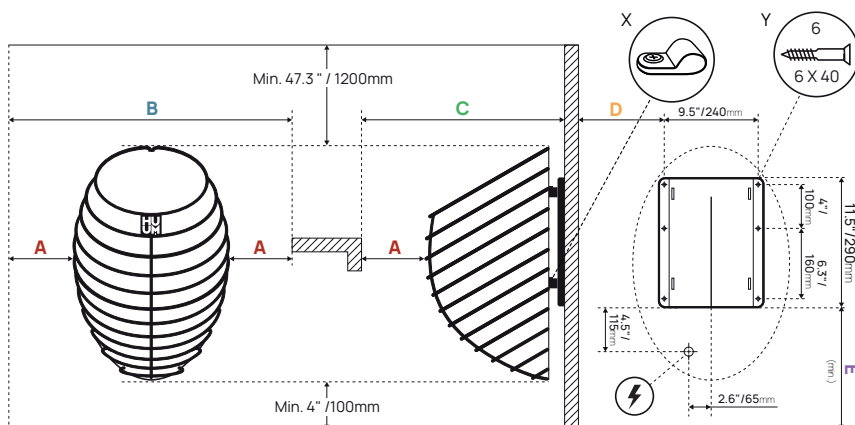
Figure 1. Montage du poêle
