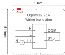
Fig. 1.110-240 V~ Power supply Abb. 1. 110-240 V~ Stromversorgung Fig. 1. Alimentazione 110-240 V~
