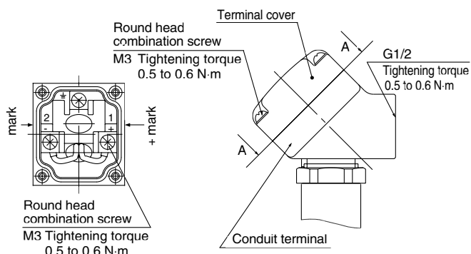
View A-A
