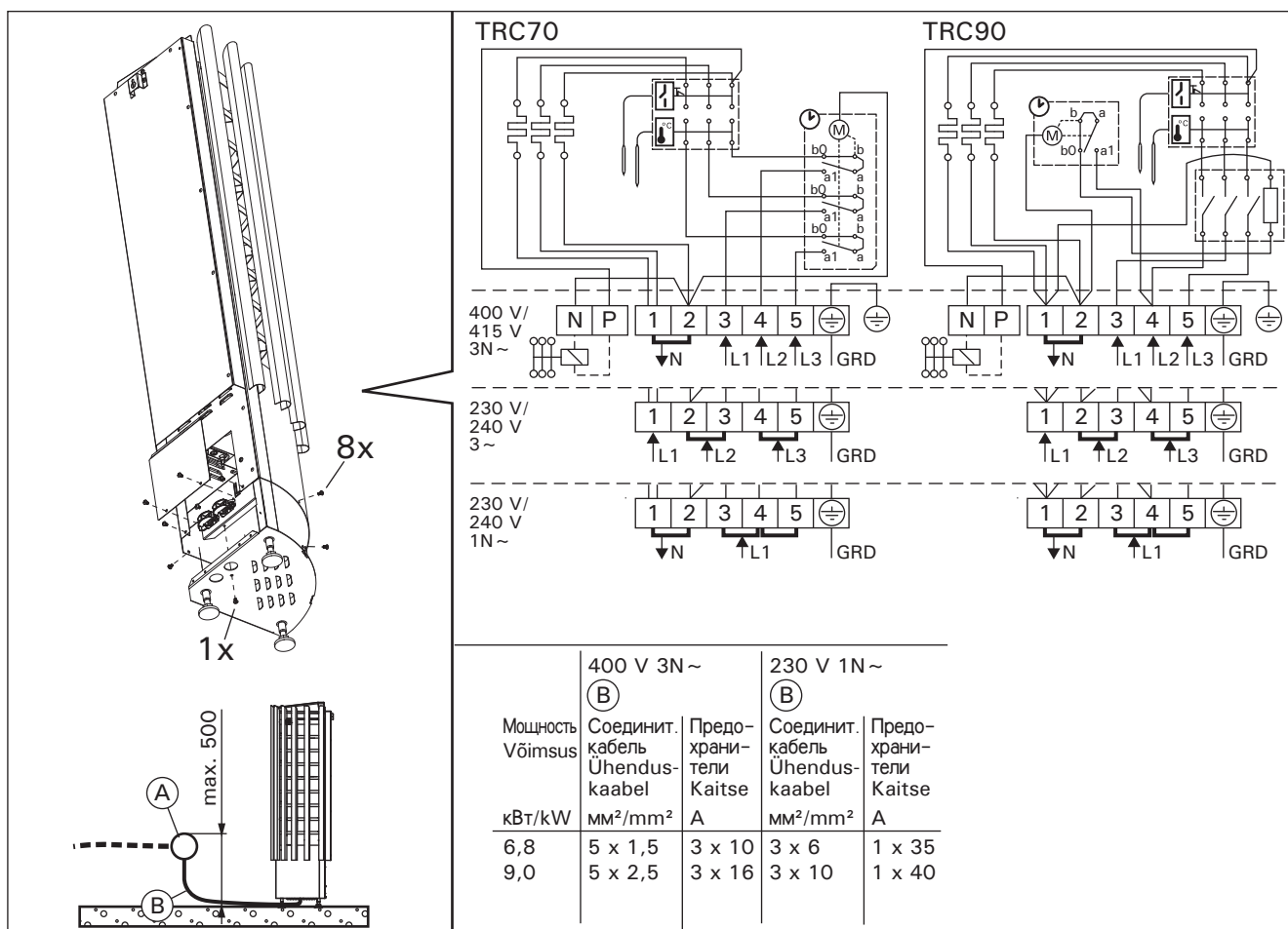
Рисунок 7. Электромонтаж Joonis 7. Elektriihendused
