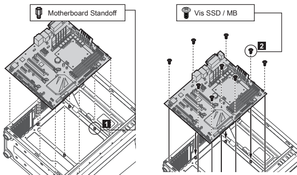
1) ATX
