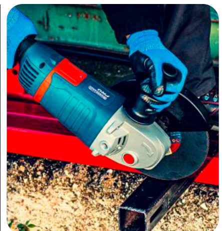
Angle grinder • 2200W • Ø230mm • 6500rpm
