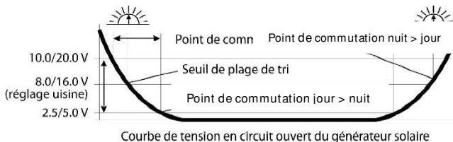
Courbe de tension en circuit ouvert du générateur solaire
