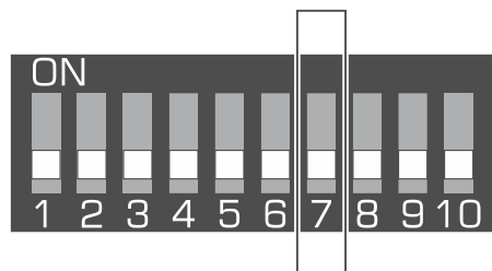
Abb. 4. Schalter zur Einschaltung / Ausschaltung der Unterstützung des nicht registrierten Testers ARF-200.
