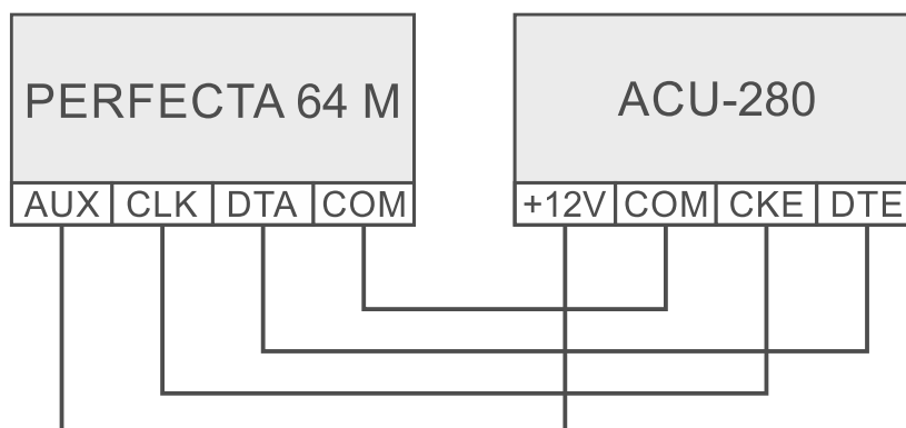
Abb. 9. Anschluss des Funkbasismoduls an die Zentrale PERFECTA 64 M.
