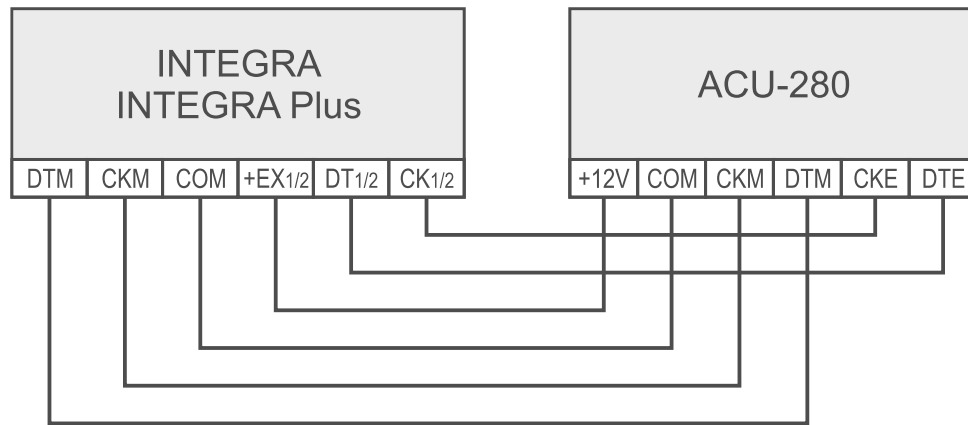
Abb. 7. Anschluss des Funkbasismoduls an die Zentrale der Serie INTEGRA.
