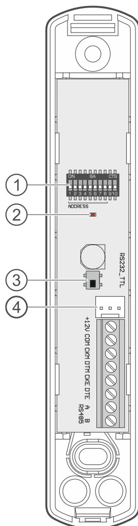
Abb. 1. Elektronikplatine des Funkbasismoduls.
