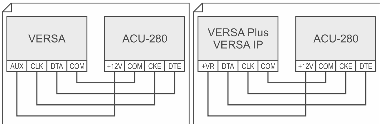
Abb. 8. Anschluss des Funkbasismoduls an die Zentrale der Serie VERSA.
