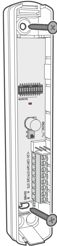
Abb. 6. Montage des Gehäuseunterteils.
