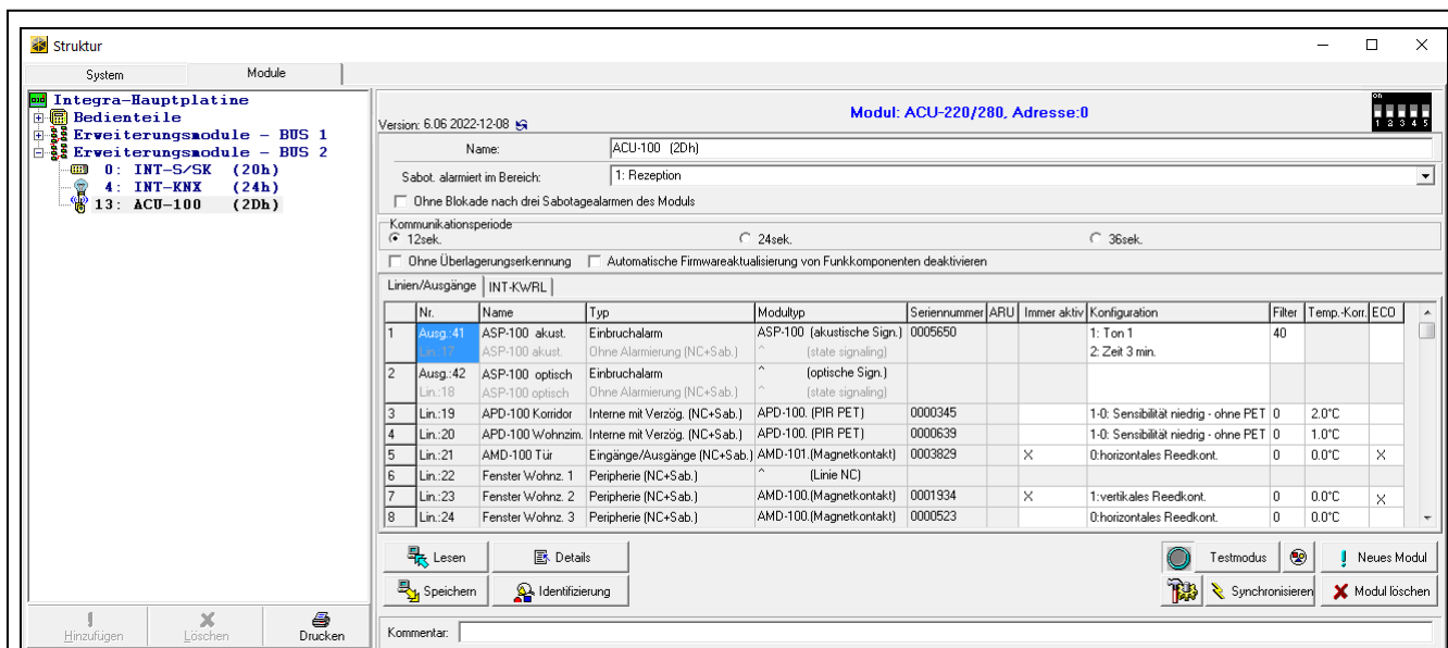
Abb. 24. Programm DLOADX: Einstellungen des Funkbasismoduls im System INTEGRA.
