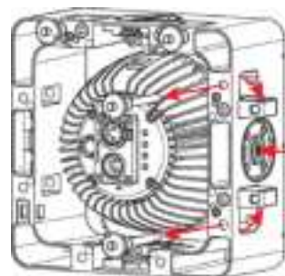
Goupille d'alignement
