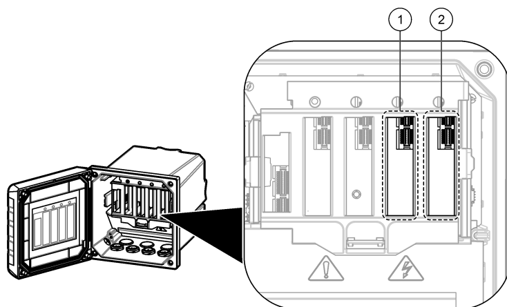
Figura 2 Ranuras para módulos de entrada de mA
