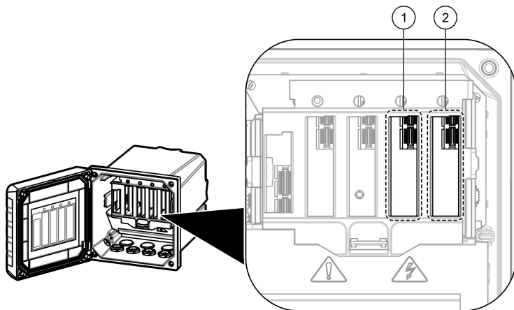
1 模拟模块插槽 — 通道 1
