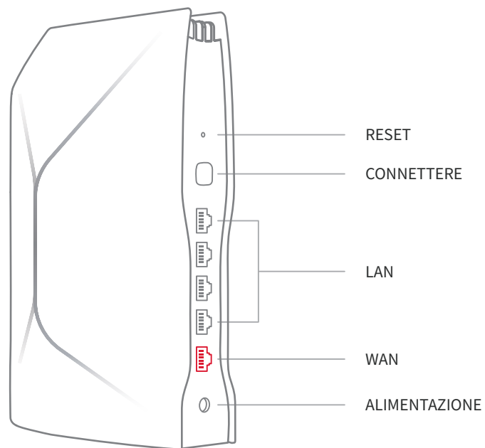
Configurazione porte
