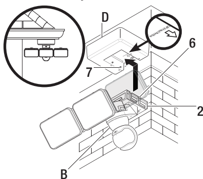
Montaje en alero
