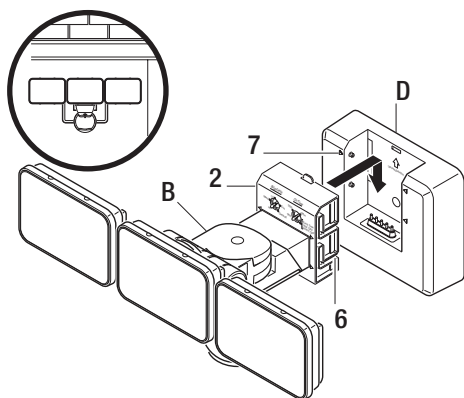
Montaje en pared
