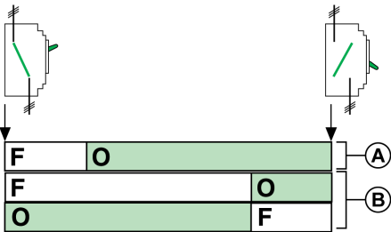
OF 指示触点与主触点关系的次序图
