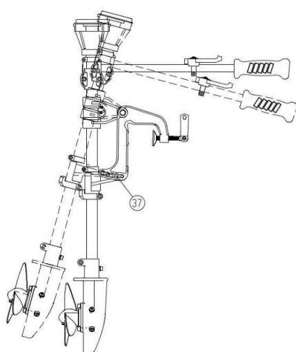
Slăbiți șurubul nr.37 pentru a regla înclinarea
