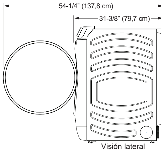
Visión lateral
