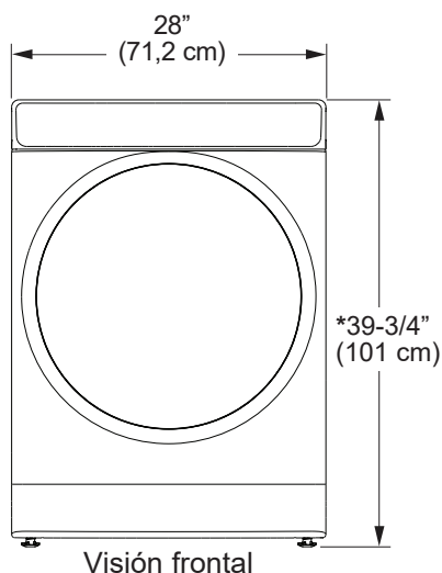
Visión frontal
