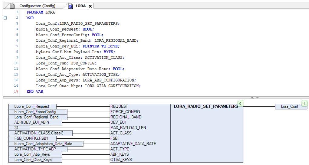
Figure 11: LORA_RADIO_SET_PARAMETERS
