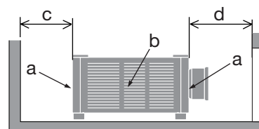
a: Nasávací vetrací otvor/b: Výstupný vetrací otvor/ c: 20 cm/8" alebo viac/d: 30 cm/12" alebo viac
