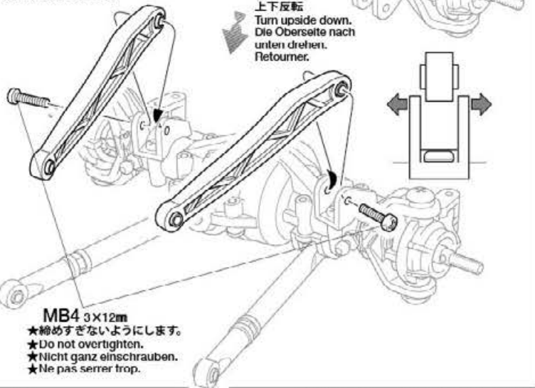
MB4 3×12mm ★締めすぎないようにします。 ★Do not overtighten. ★Nicht ganz einschrauben. ★Ne pas serrer trop.
