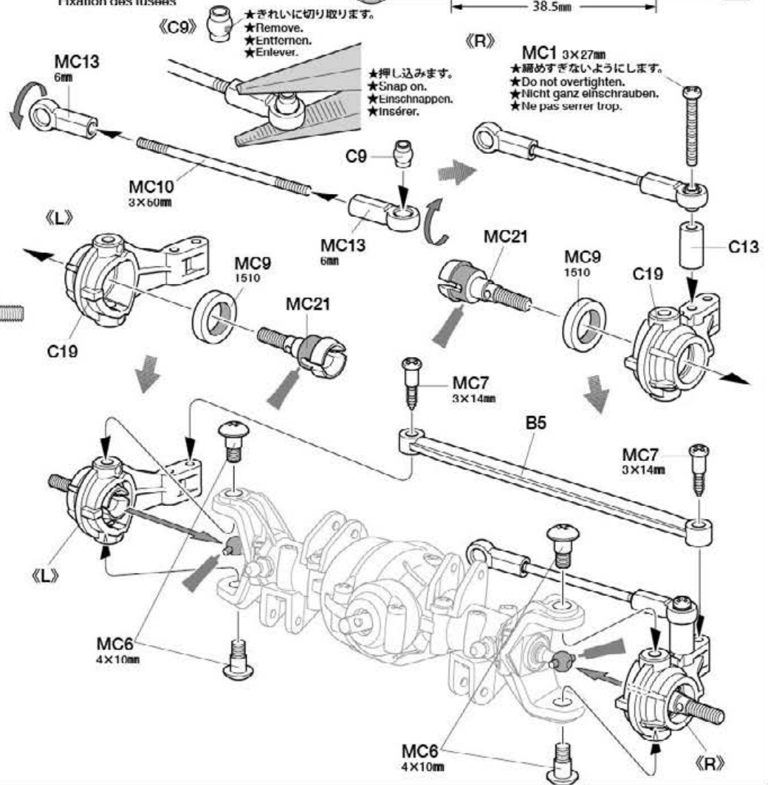
MC7 x2 3×14mm段付タッピングビス Step screw Paßschraube Vis décollée
