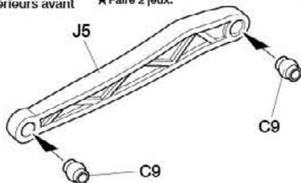
《フロントロウアーム》 Front lower arms Vordere, untere Lenker Tirants inférieurs avant
