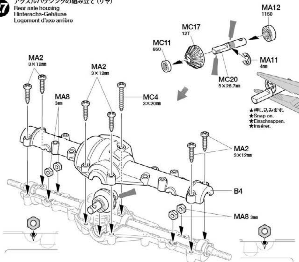
MA12 x1 1150 プラベアリング Plastic bearing Plastik-Lager Palier en plastique
