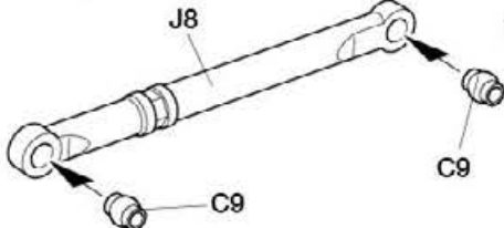
《フロントロウアーム》 Front lower arms Vordere, untere Lenker Tirants inférieurs avant
