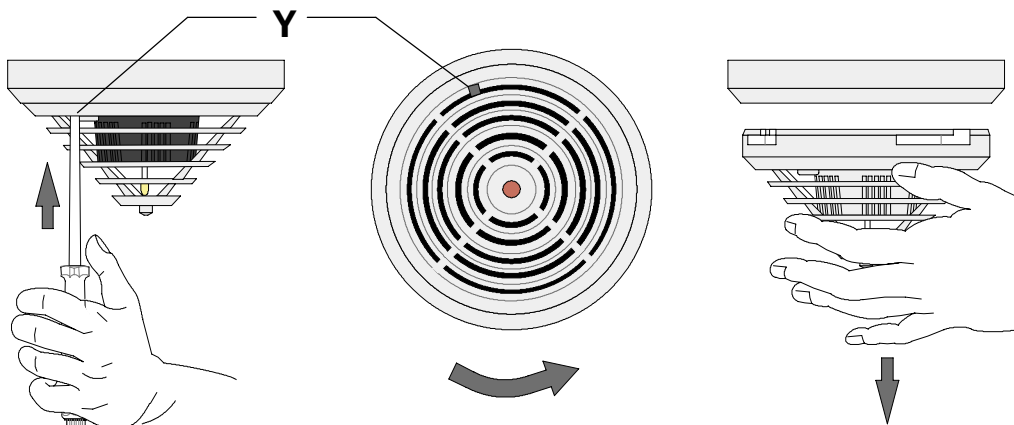
Abbildung 5.2: Melderentnahme (verriegelter Meldereinsatz)
