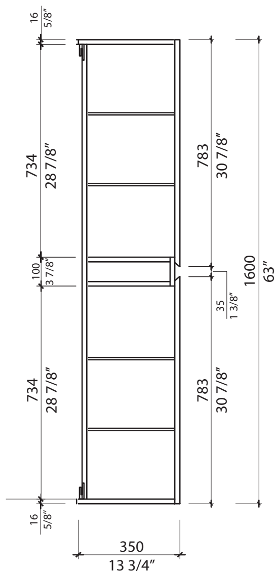
Élévation latérale Side elevation
