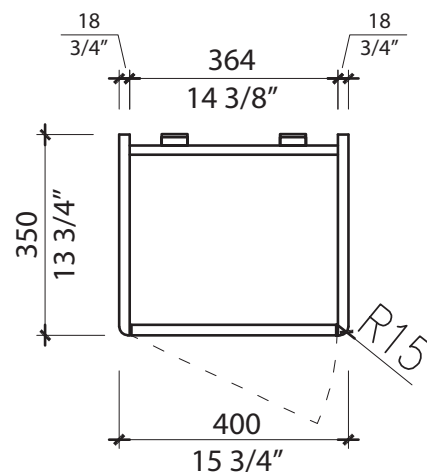
Vu de dessus Top view
