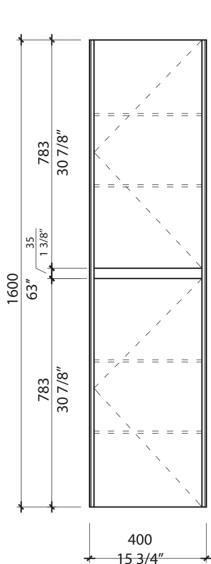
Vu de devant Front view
