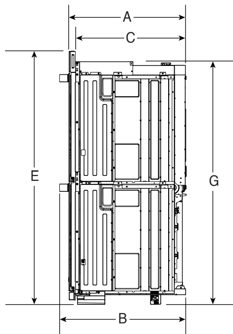
VUE LATÉRALE
