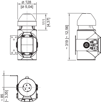
Bocina omnidireccional YA60/3
