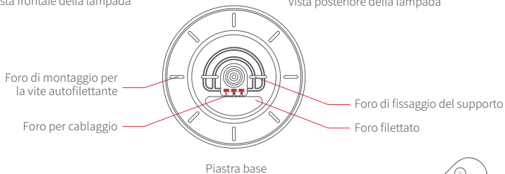
Piastra base
