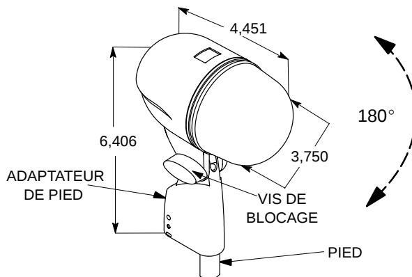
ADAPTATEUR DE PIED INTÉGRAL BETA 52A FIGURE 3
