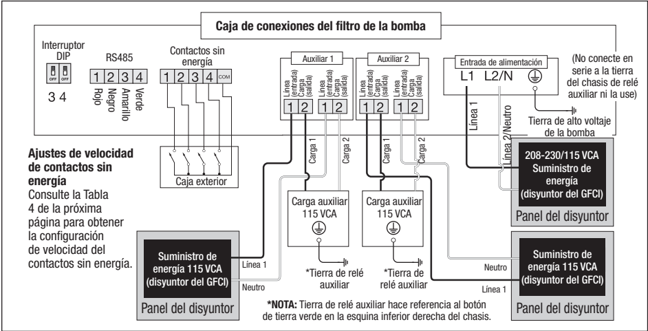
Figura 13. Diagrama de cableado de relé auxiliar de 115 V*
