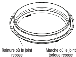
Figure 16. Installation du joint torique test de pression bleu
