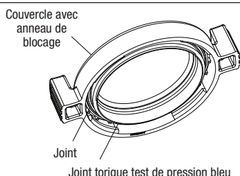
Figure 14. Joint torique test de pression bleu
