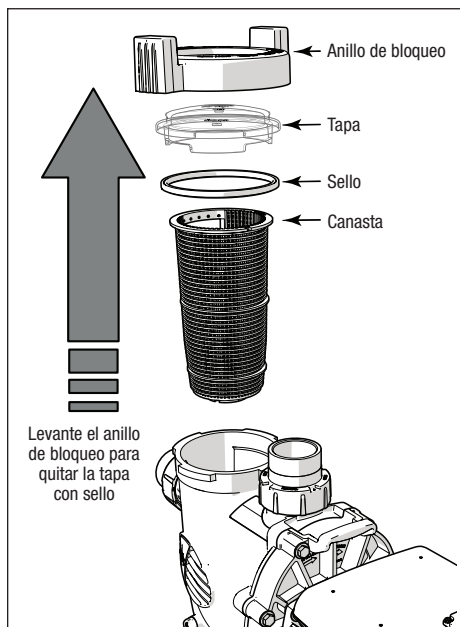
Figura 18. Quitar la tapa de la bomba
