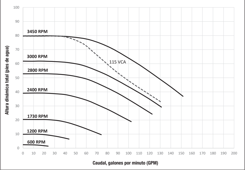
Curvas de desempeño de VSSHP220DV2A(S)
