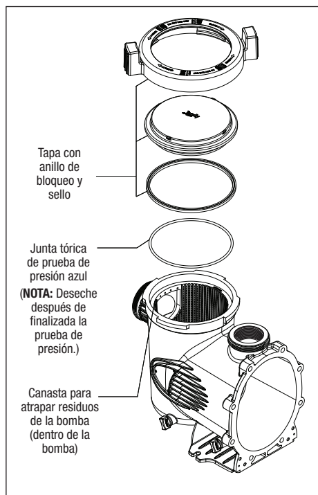
Figura 15. Vista ampliada con junta tórica de prueba de presión azul (modelos de bomba VSSHP únicamente)
