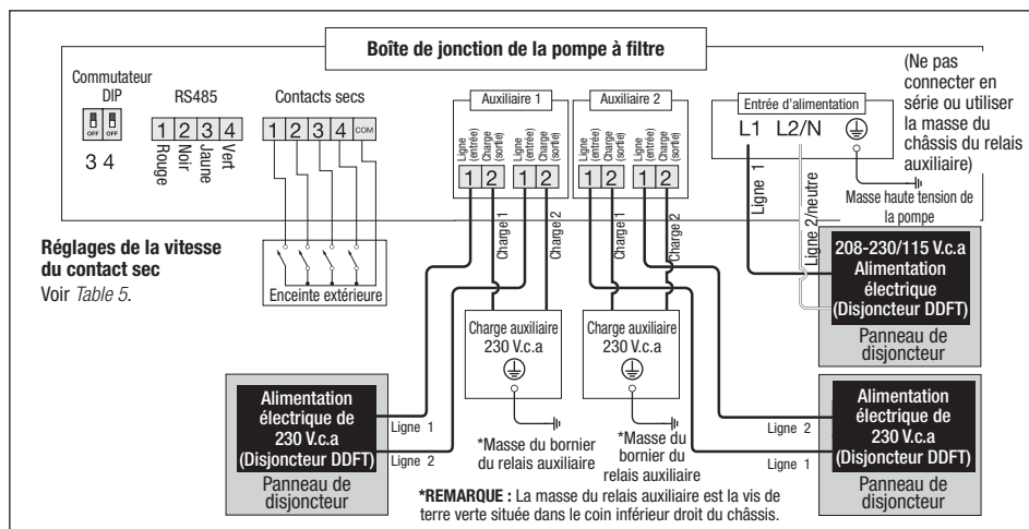
Figure 12. Schéma de câblage du relais auxiliaire de 208-230 V*
