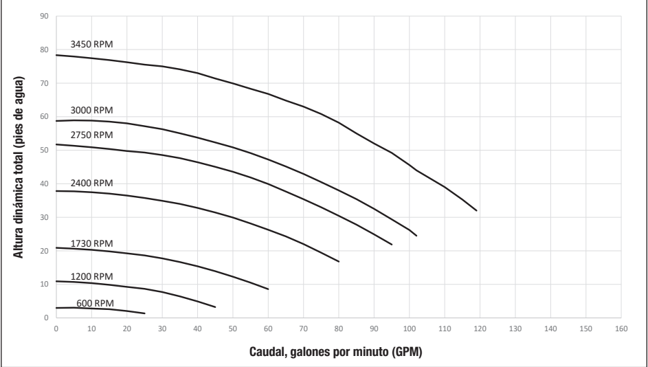
Curvas de desempeño de VSFHP185DV2A(S)
