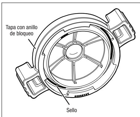
Figura 17. Junta tórica en el conjunto de la tapa
