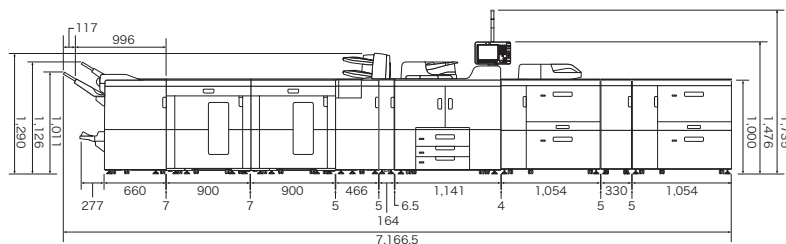
RICOH Pro 8120S/8110S/8100S 価格表 外形寸法
