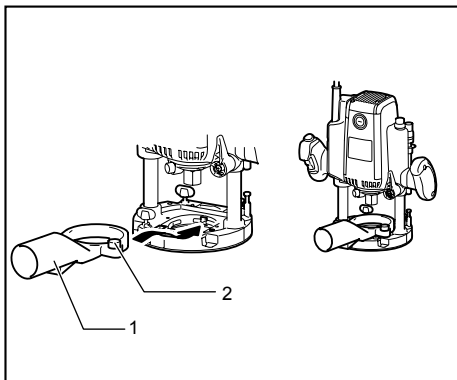
1. Porkifúvó 2. Szorítócsavar
