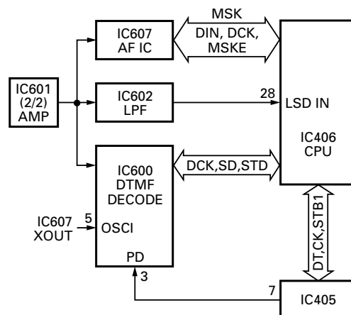
Fig. 16 Decode
