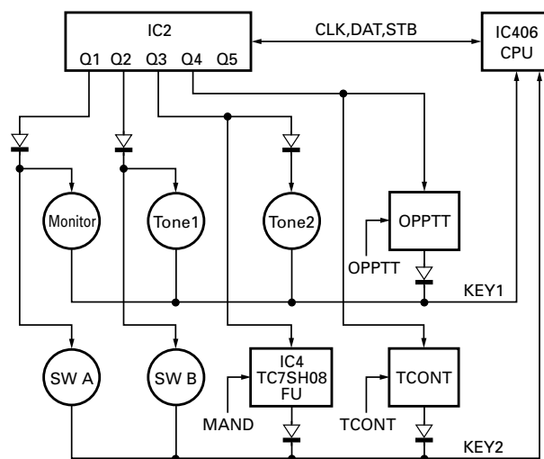
Fig. 14 Key input
