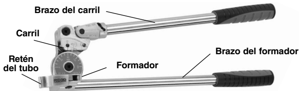
Figura 1 – Doblatubos serie 600
