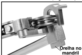
Figura 2 – Ponto de montagem no mandril
