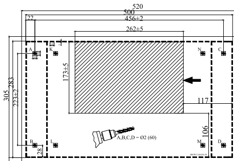
Фигура 3 - Монтажен шаблон
