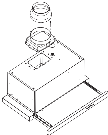
Фигура 4 - Монтаж на възвратна клапа и адаптора
