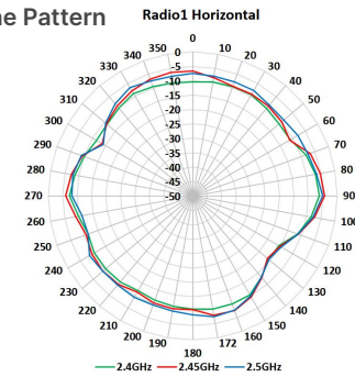
H-Plane Pattern
