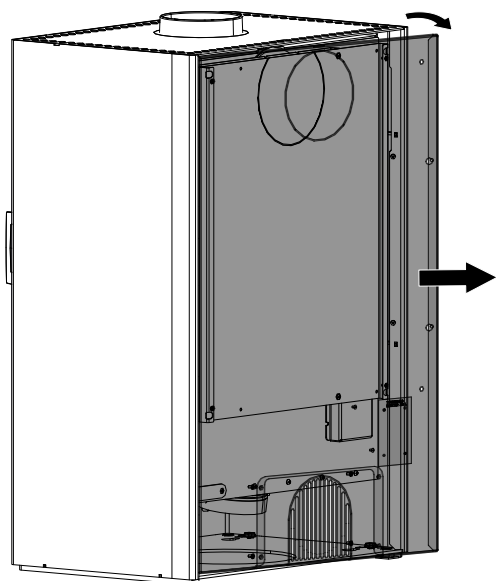
Fig. 40: Décrocher la paroi arrière
