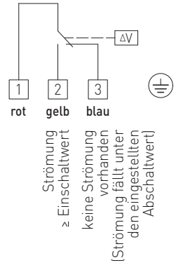
Schaltbild
