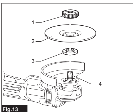
► 1. Ezynut 2. Abrasive wheel 3. Inner flange 4. Spindle
