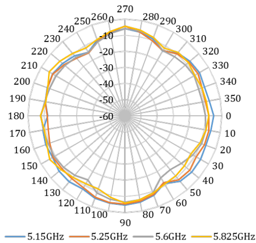
Radio2 Horizontal
